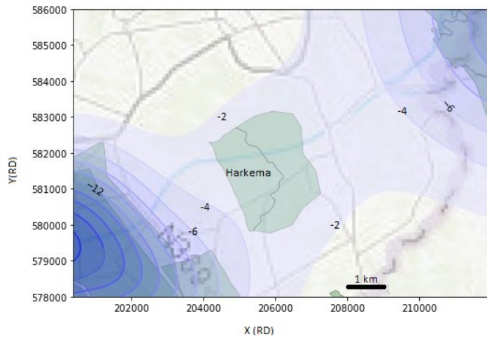
Figuur 1 controleberekening samengestelde bodemdaling
