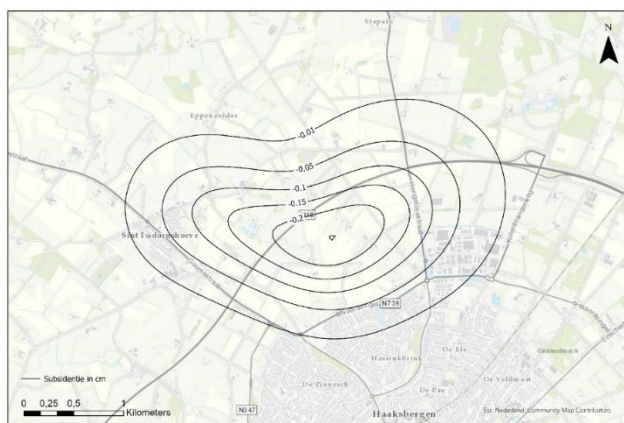
Figuur 3-1: Verwachte bodemdaling 50 jaar na start productie (in m.) voor 12 cavernes met een veilige omvang van gemiddeld 2,1 miljoen m 3 .
