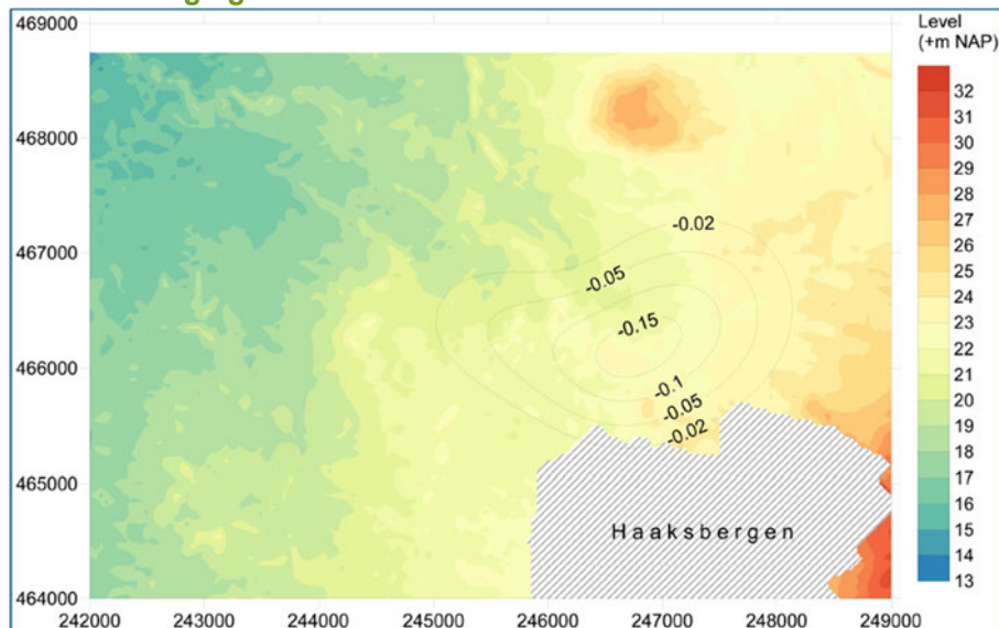
Figuur 6-1: Verwachte bodemdaling na 20 jaar, 12 cavernes van 2,1 miljoen m 3 .
