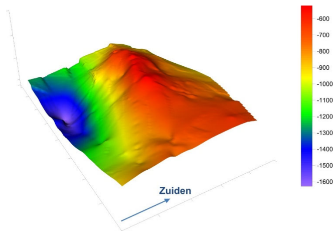
Figuur 2-1: Geologisch model met top van het zoutkussen.
