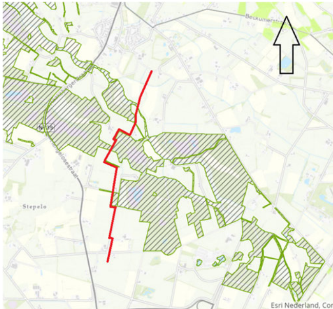
Figuur 6-3: Ligging van transportleidingen (rood) door NNN (gearceerd)
