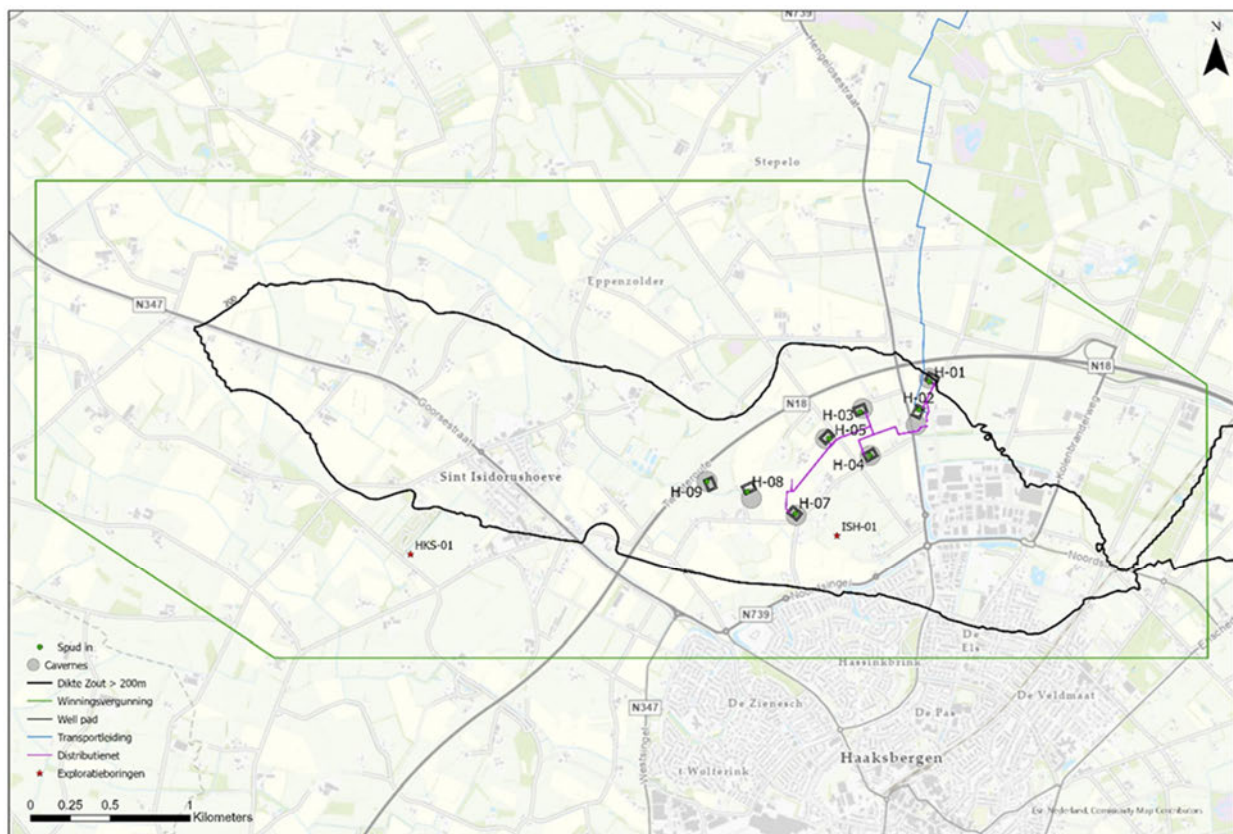
Figuur 1-2: Het projectgebied met cavernes en leidingwerk.
