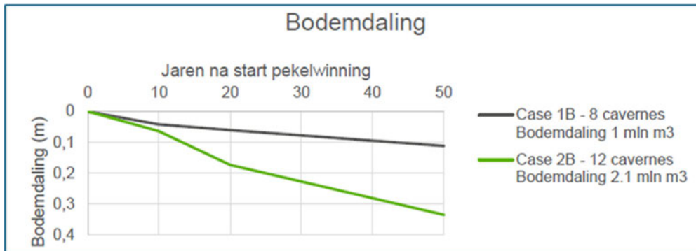
Figuur 3-2: Bodemdaling voor variant 1-B (8 cavernes) en 2-B (12 cavernes) na 50 jaar.
