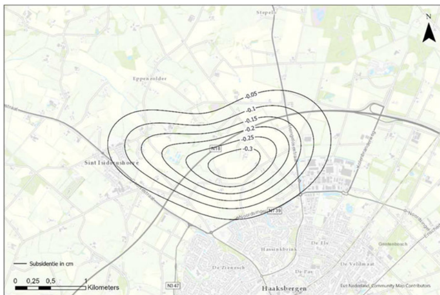
Figuur 6-2: Verwachte bodemdaling na 50 jaar, 12 cavernes van 2,1 miljoen m 3 .
