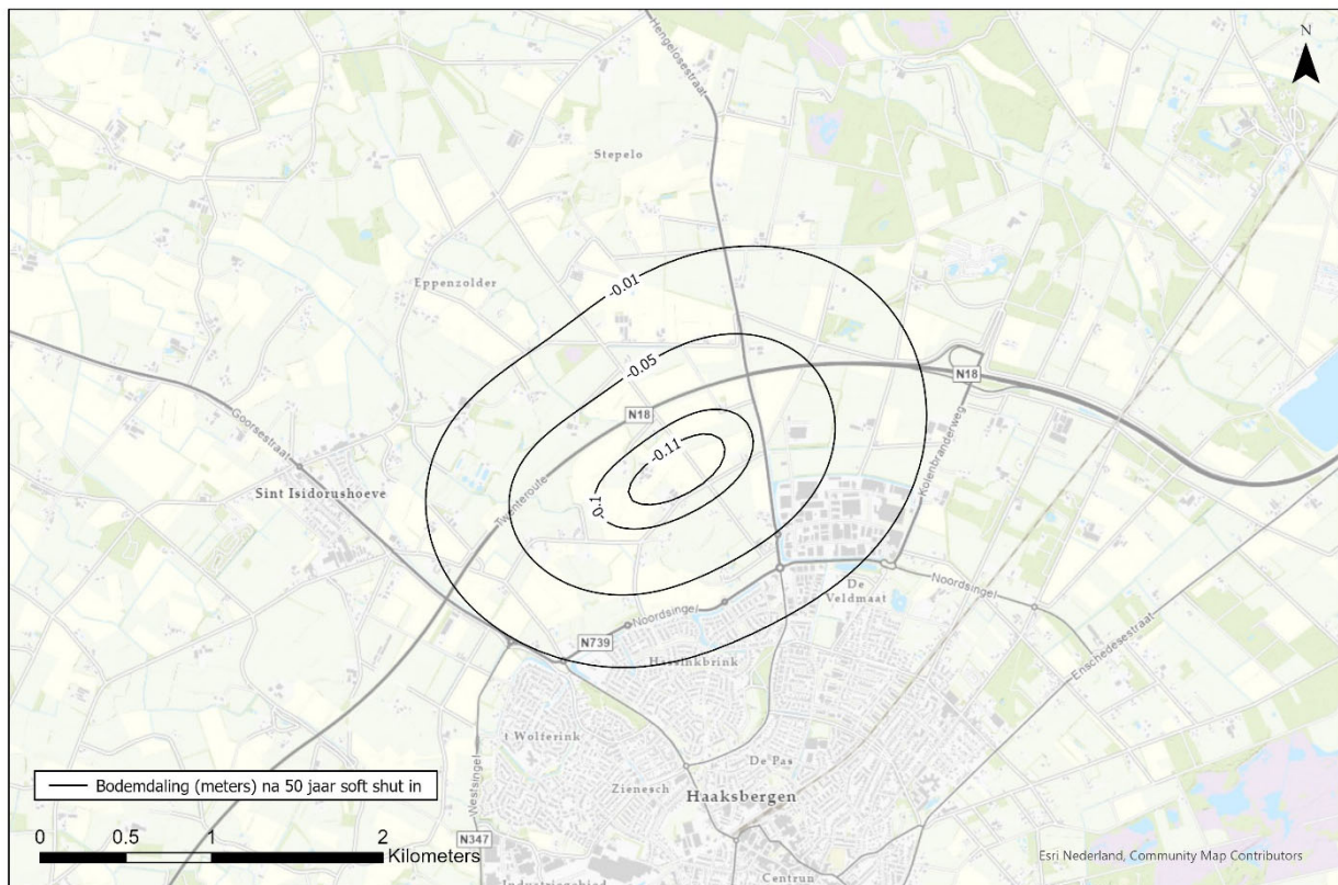
Figuur 3-3: Bodemdaling voor het feitelijke project: 8 cavernes van 1 miljoen kubieke meter na 50 jaar.
